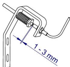
Betriebsstellung
